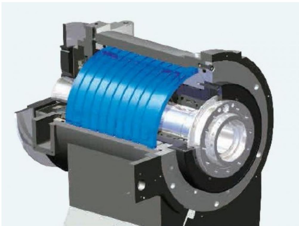
Elettromandrino con trasmissione diretta
