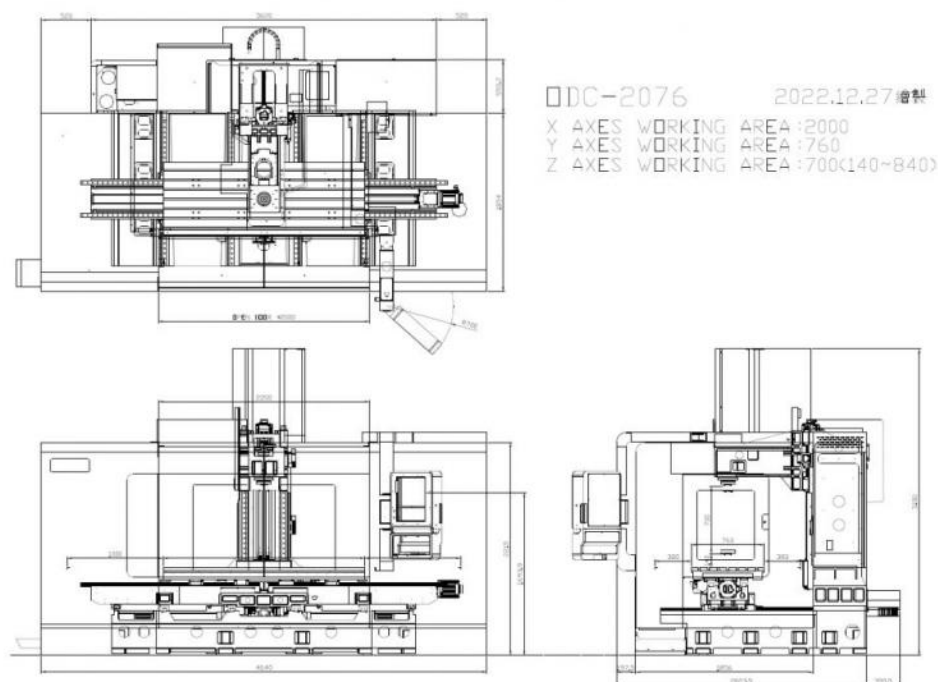
Layout macchina
