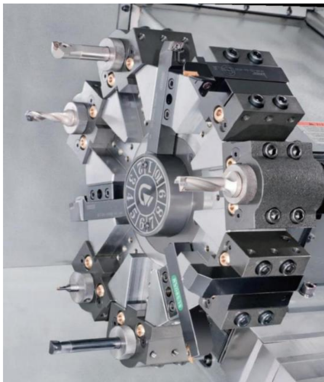
Torretta 12 posizioni
