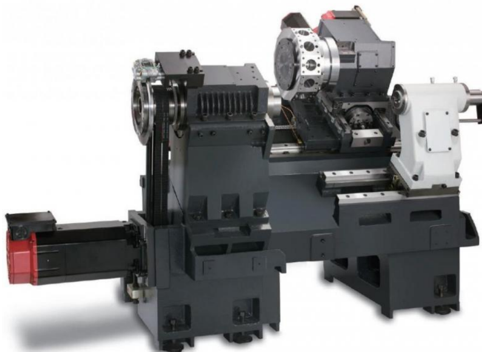
Struttura su guide a rulli
