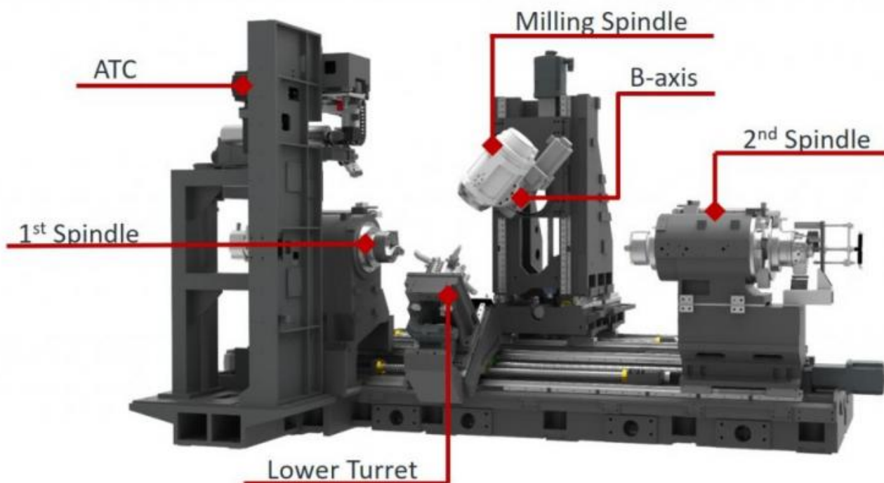
Struttura macchina
