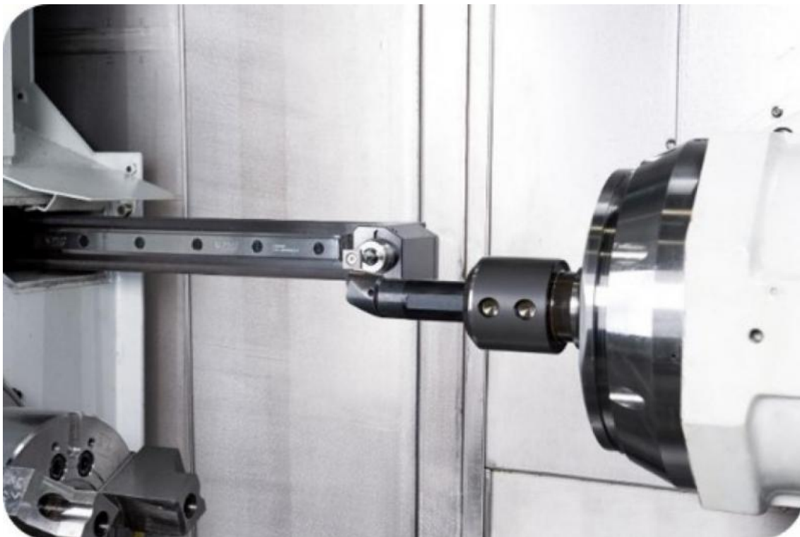
Presetting automatico Renishaw
