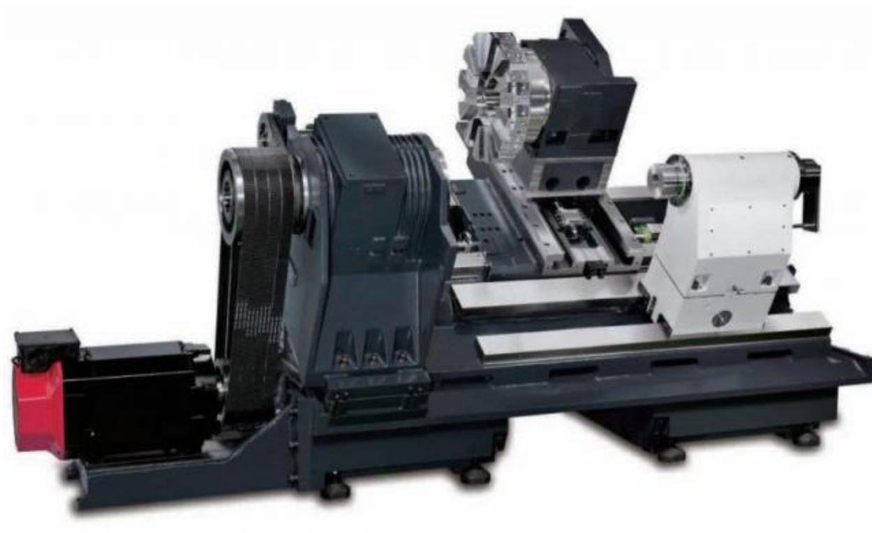
Struttura macchina su guide piane
