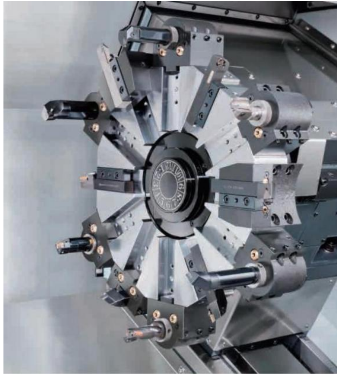
Torretta a 12 posizioni
