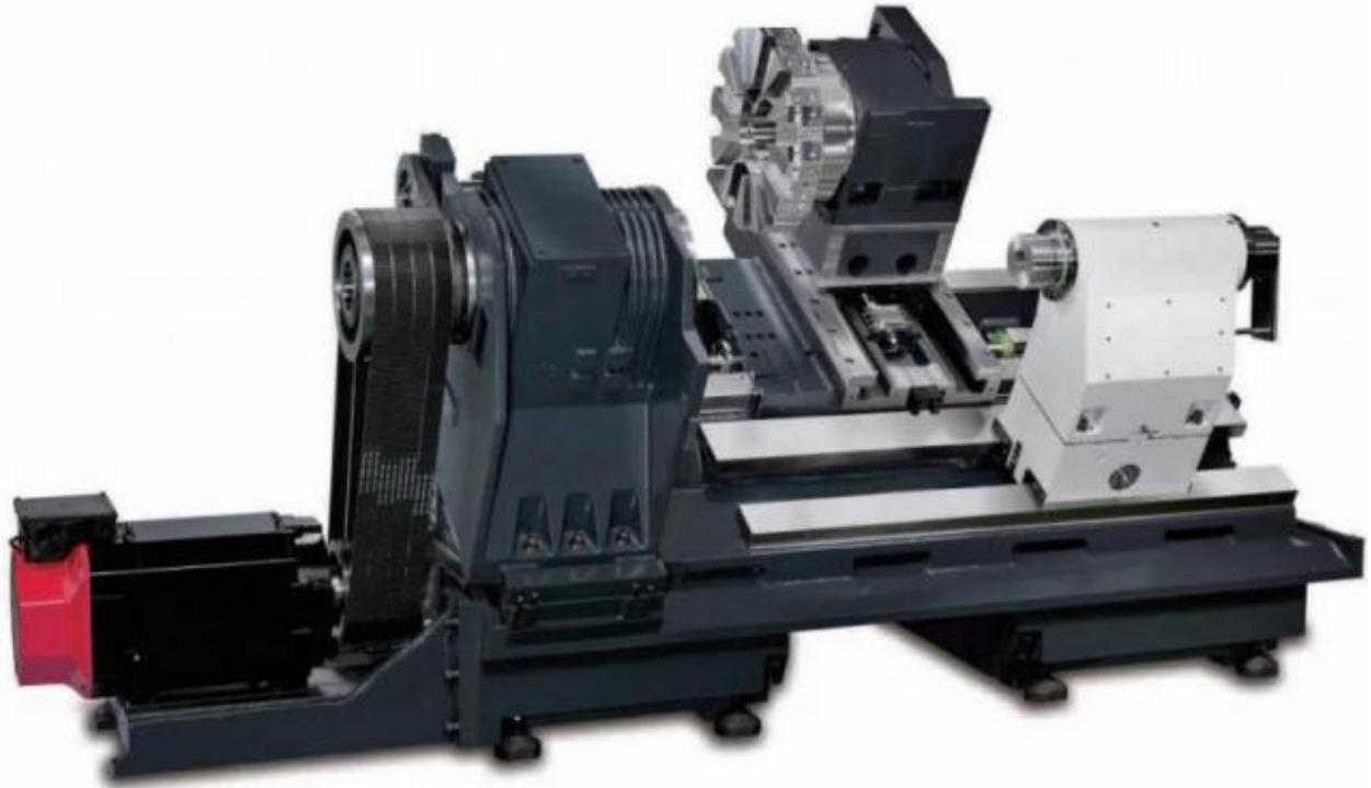
Struttura macchina su guide piane
