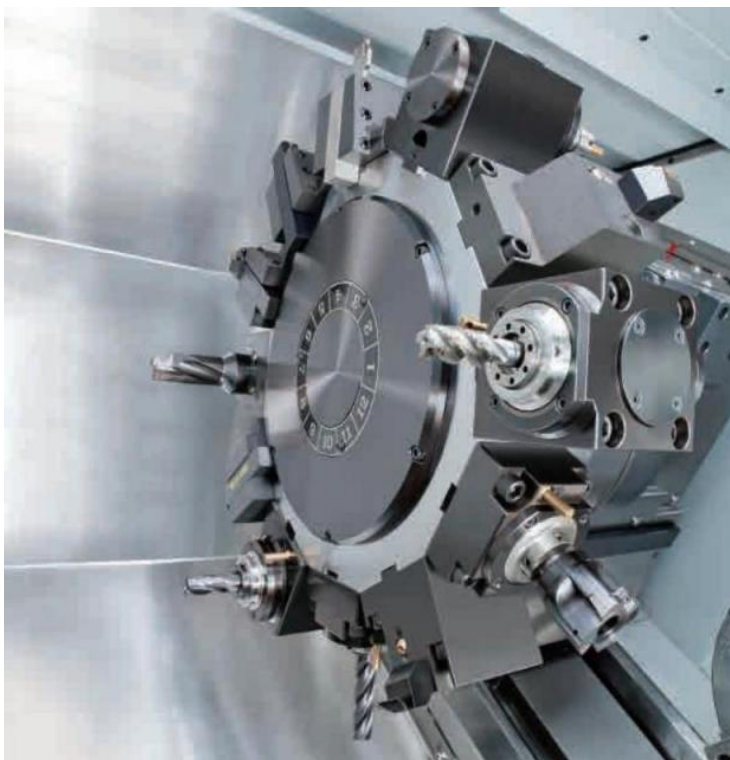
Torretta motorizzata a 12 posizioni (OPZ.16 pos.)
