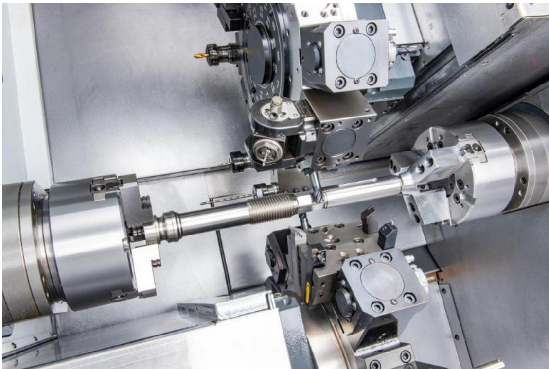
Mandrino e contromandrino speculari
