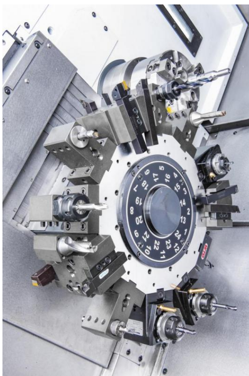
Doppia torretta 12 posizioni
