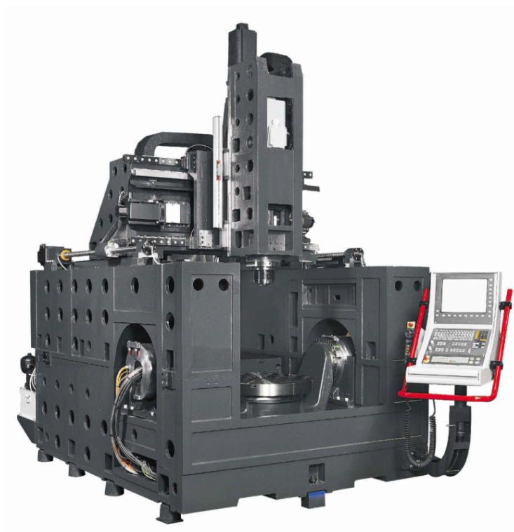
Struttura macchina su guide a rulli
