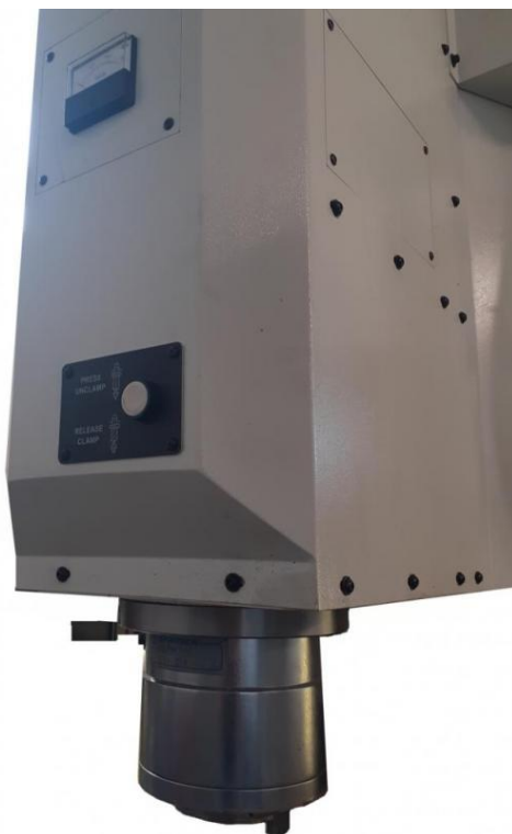
Linea mandrino SPINDER ISO40 - RPM 6.000 - HP10
