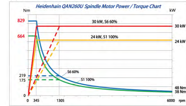
(2) Heidenhain QAN260U, 24/30kW, 6000rpm
