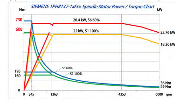
(2) SIEMENS 1PH8137-1xFxx, 22/26.4kW, 6000rpm
