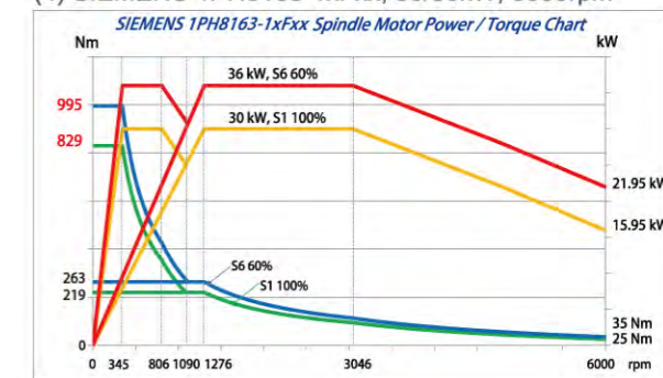
(4) SIEMENS 1PH8163-1xFxx, 30/36kW, 6000rpm
