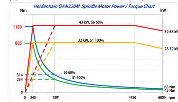
(4) Heidenhain QAN320M, 32/43kW, 6000rpm
